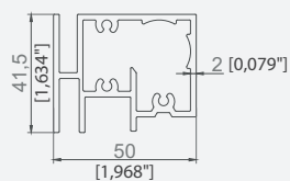
PROFIL MONTANT CU PISTON
