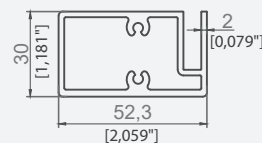
PROFIL INFERIOR PANOU DIN STICLĂ
