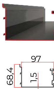
④ PROFIL JGHEAB
