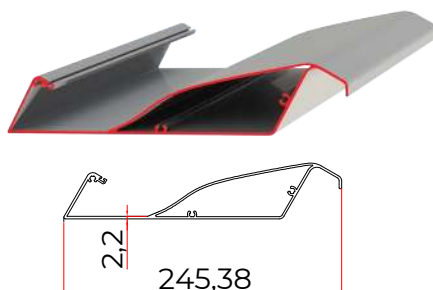
⑦ PROFIL DE LAMELĂ
