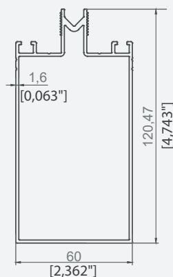
PROFIL SUPT STICLĂ STANDARD
