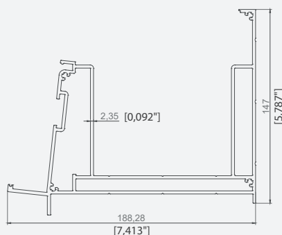
PROFIL JGHEAB DREPT 188,28X147
