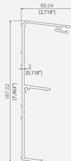
PROFIL TRAVERSĂ POSTERIOARĂ 69X187
