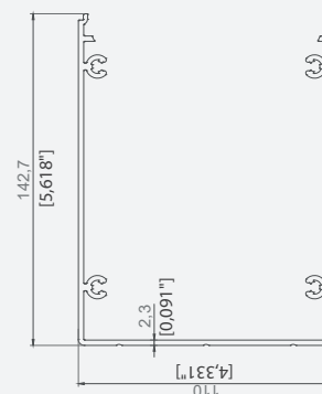
PROFIL CORP STĂLP 110x142,7
