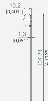
CAPAC JGHEAB ȘI TRAVERSĂ POSTERIOARĂ 10,2X104,71
