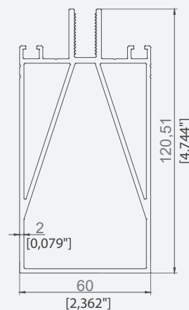
PROFIL SUPT STICLĂ RANFORSAT
