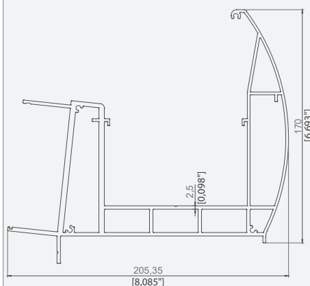
PROFIL JGHEAB OVAL 205X170
