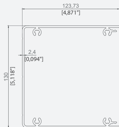
PROFIL CORP STÂLP 123x130
