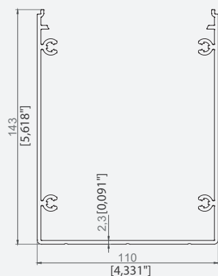
PROFIL CORP STALP 110x142,7
