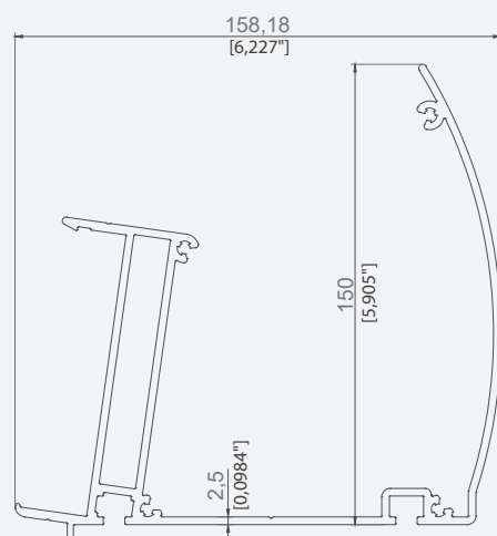
PROFIL JGHEAB OVAL 158X150
