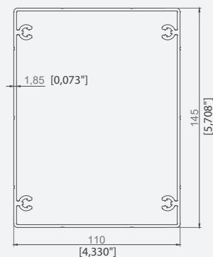
PROFIL STĂLP 110X145
