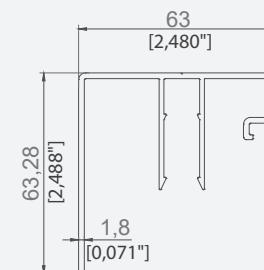
PROFIL CAPAC LATERAL STICLĂ 63X63,2
