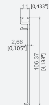
CAPAC JGHEAB ȘI TRAVERSĂ POSTERIOARĂ 11X106,37
