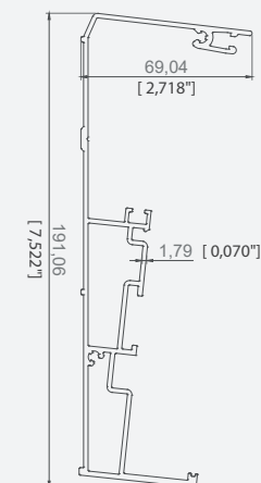
PROFIL TRAVERSĂ POSTERIOARĂ 69X191
