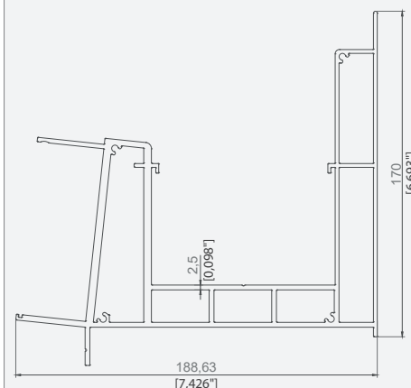
PROFIL JGHEAB DREPT 188X170
