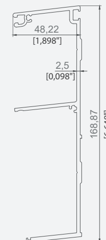
PROFIL TRAVERSĂ POSTERIOARĂ
