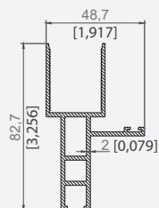
PROFIL DE ANTRENARE PANOU
