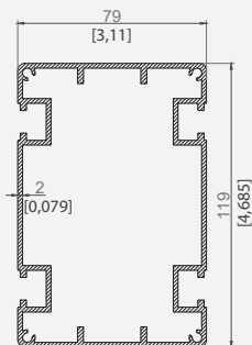
PROFIL PORTANT
