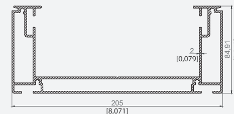
PROFIL JGHEAB
