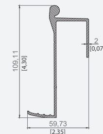
PROFIL DE LEGĂTURĂ ȘINĂ - JGHEAB
