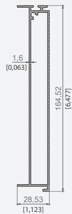
PROFIL DE PRELUNGIRE JGHEAB
