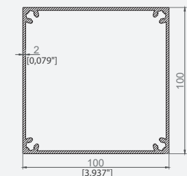
PROFIL STÂLP
