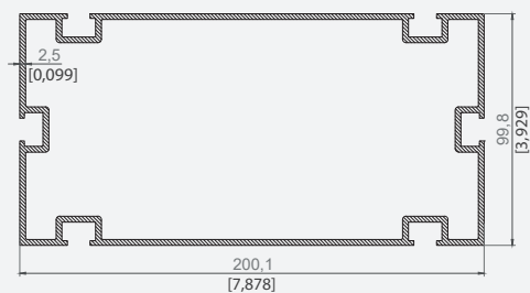
PROFIL GRINDĂ SPATE
