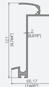
PROFIL ȘINĂ REGLABILĂ
